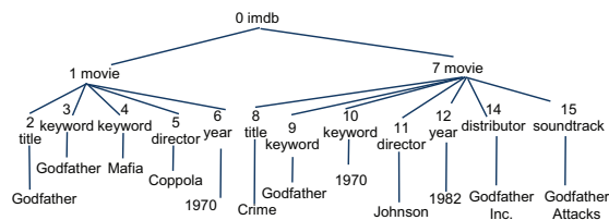
Fig. 1. IMDB database fragment.
